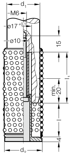
Einbaubeispiel
