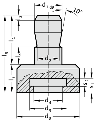
212.16. Aufnahmefutter für Kupplungsaufen
