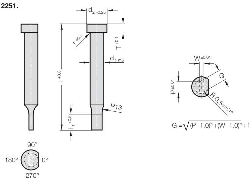
2251. Schneidstempel, abgesetzt, Rechteck mit Radius, ISO 8020
