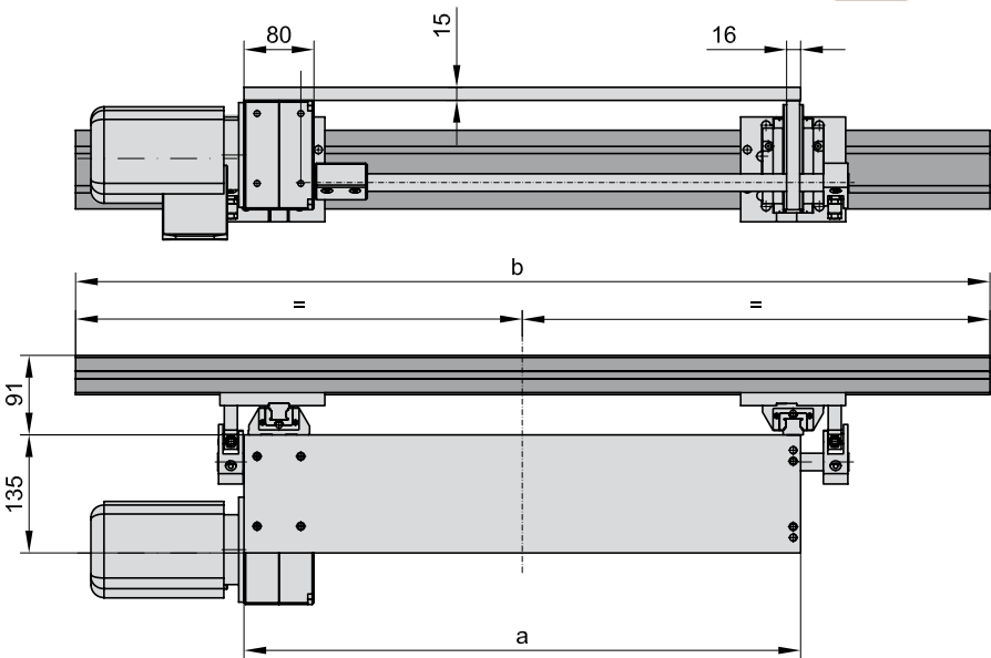
2299.121. vertikale Getriebelage, 2 Schlitten, mit Profil und Träger
