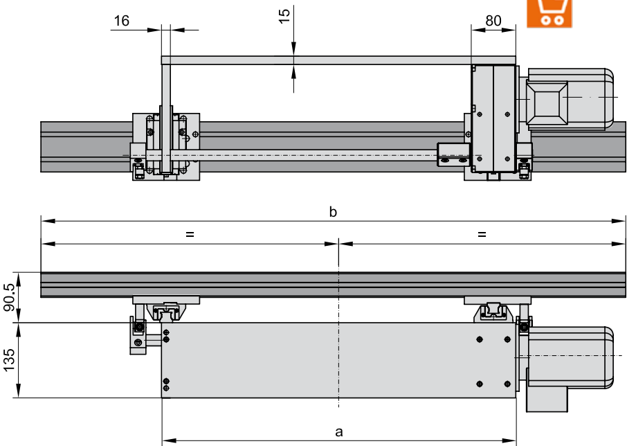
2299.122. horizontale Getriebelage, 2 Schlitten, mit Profil und Träger
