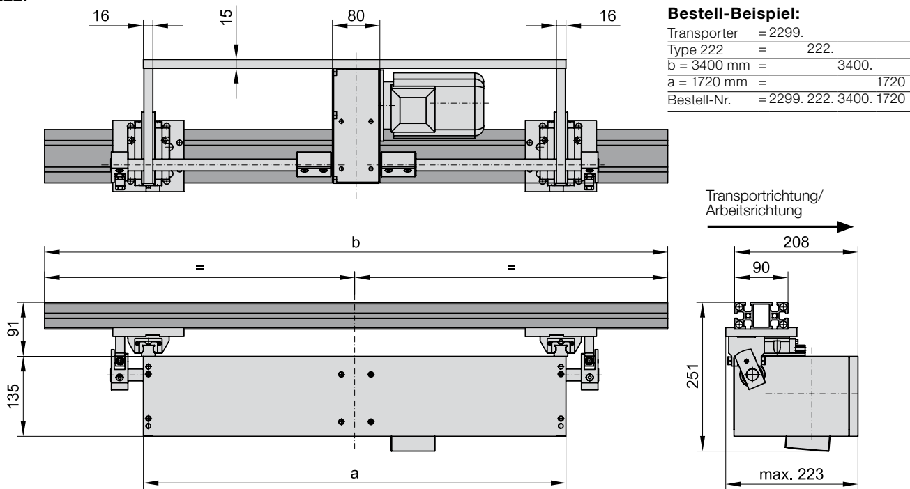
2299.222. mittig horizontale Getriebelage, 2 Schlitten, mit Profil und Träger
