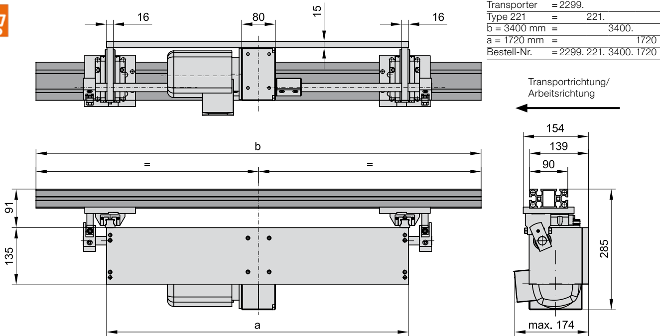
2299.221. mittig vertikale Getriebelage, 2 Schlitten, mit Profil und Träger
