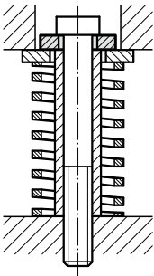
Einbaubeispiel
