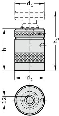
2140.20. Soporte ajustable
