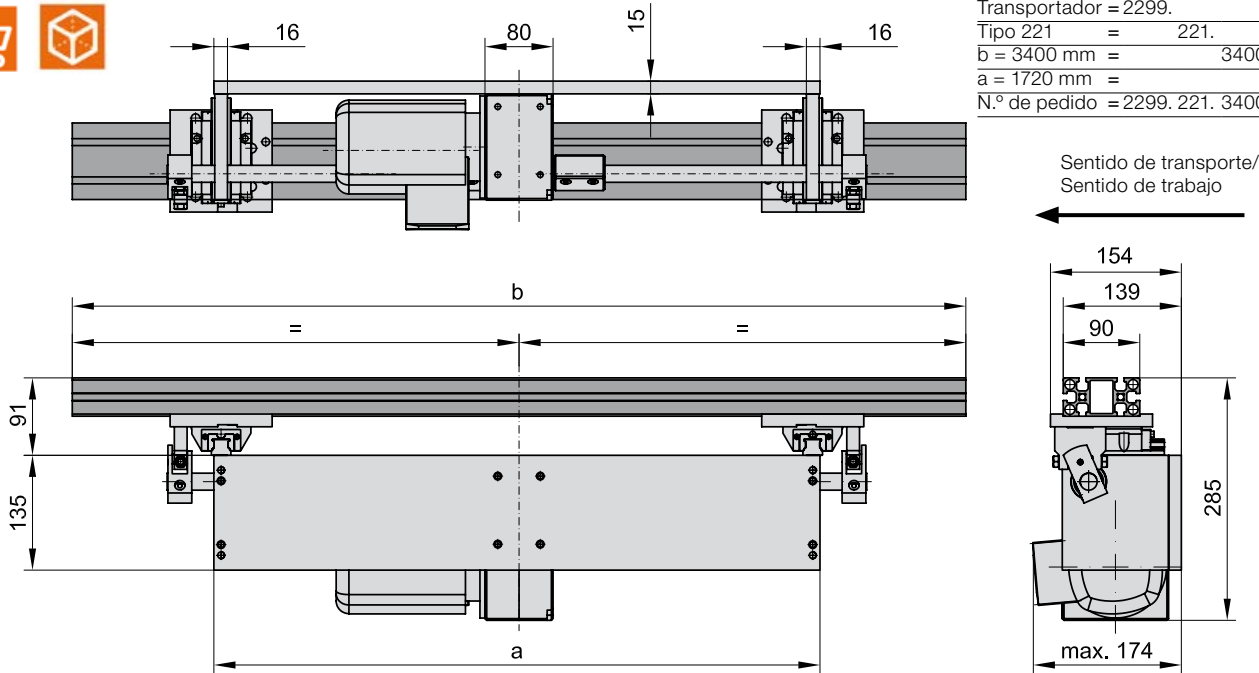
2299.221. posición de accionamiento central vertical, 2 carros, con perfil y soporte
