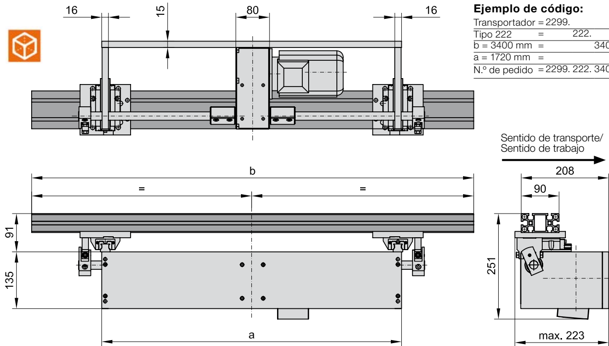
2299.222. posición de accionamiento central horizontal, 2 carros, con perfil y soporte
