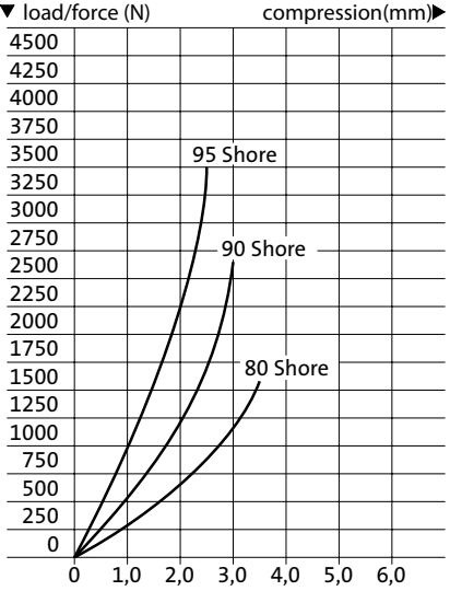
244.1.40. – ø 40
