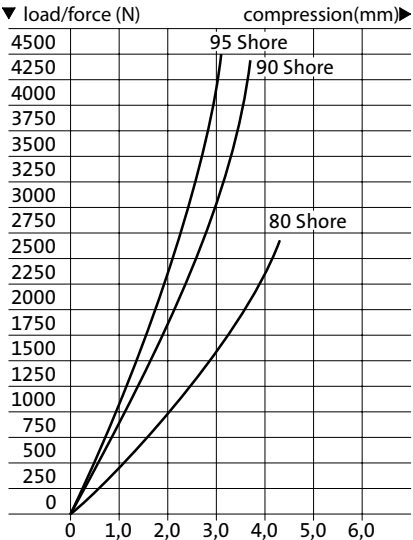
244.1.25. – ø 25
