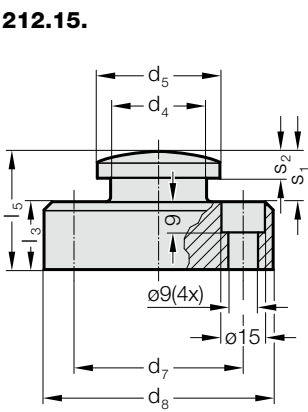
212.15. Tourillon d'accouplement fixé par vis
