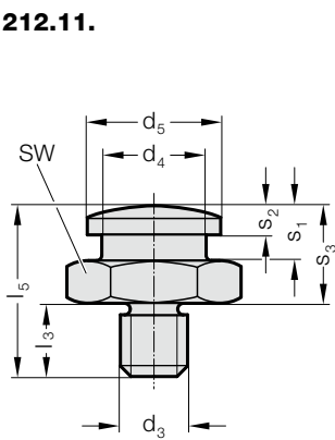
212.11. Tourillon d'accouplement avec filetage
