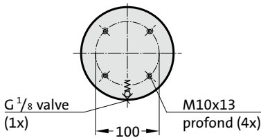
Vue selon X - Ressort à gaz
