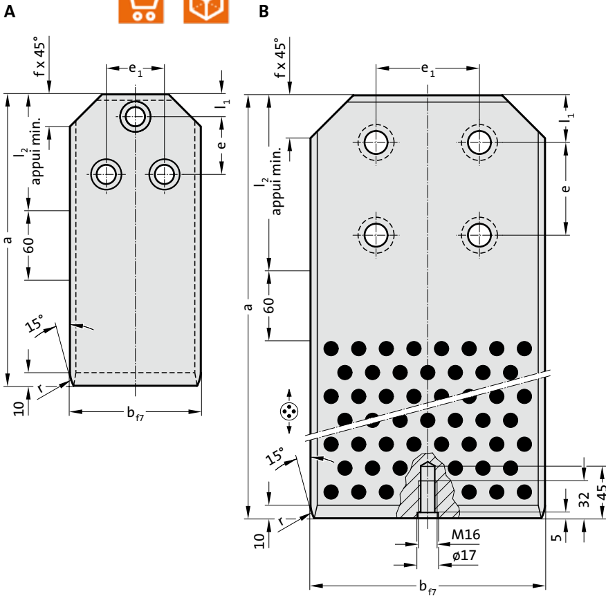
2960.89. Plaque de guidage, Bronze avec lubrifiant solide, VDI 3387
