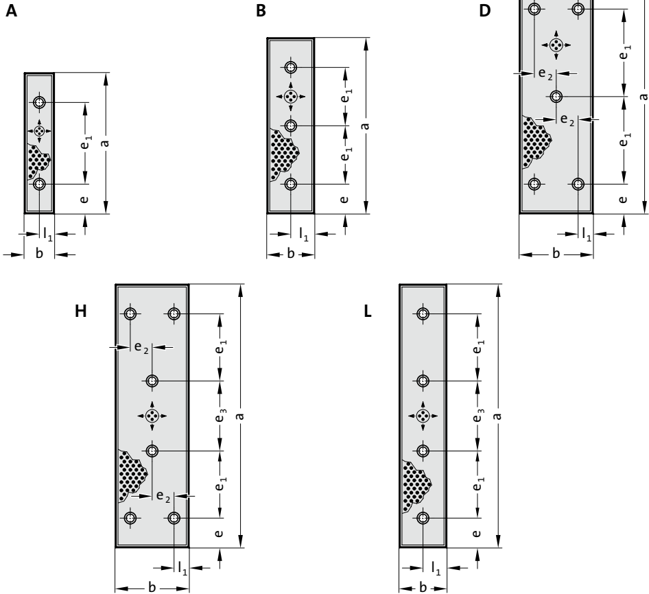
2962.85. Plaque de frottement, Acier avec lubrifiant solide
