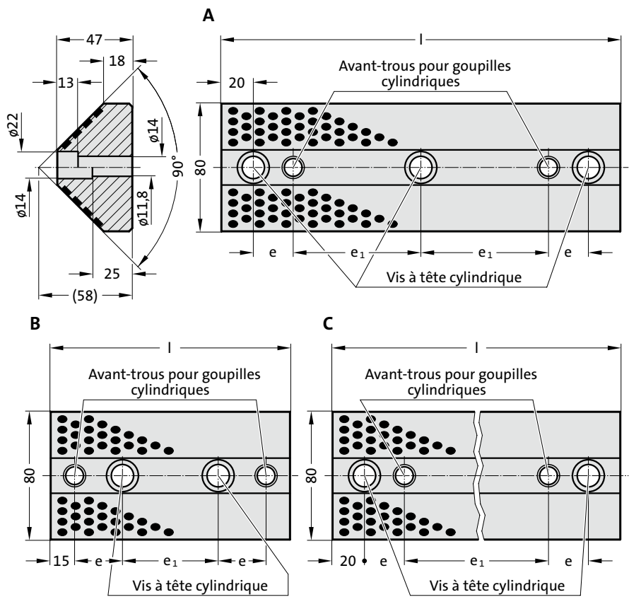
2963.80. Patin coulissant, Bronze avec lubrifiant solide
