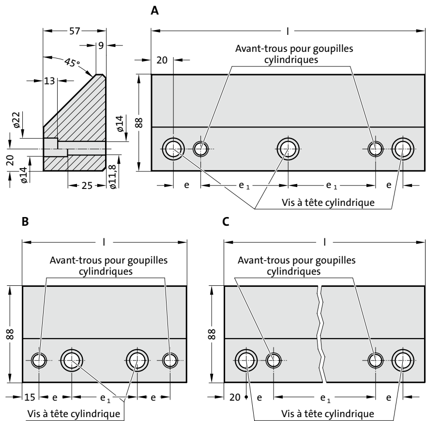
2965.82. Patin coulissant prismatique unilatéral, Acier
