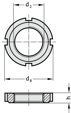
2073.48. Slotted nut DIN 1804
