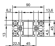
Przekrój poprzeczny profilu
